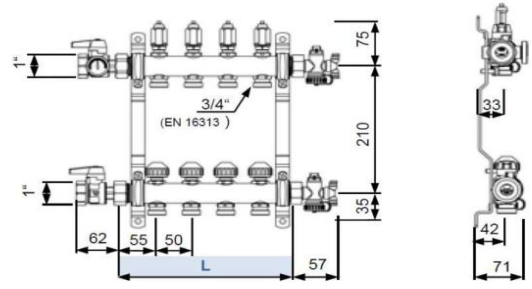
ÇELİK KOLLEKTÖR
