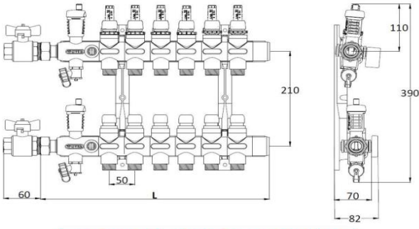
KOMPOZİT KOLLEKTÖR
